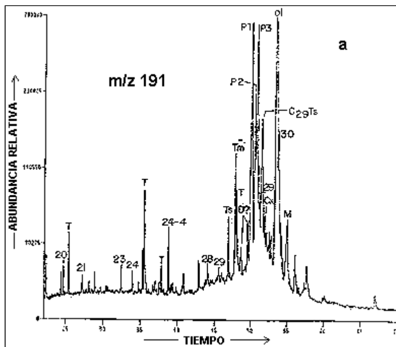
Cromatograma de la fracción saturada del mene Quirós (Tomado de: Del Olio, 1993)
