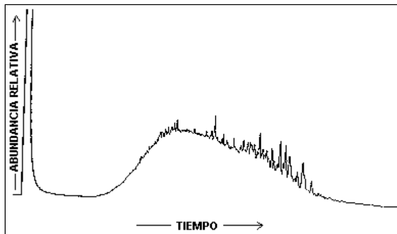
Cromatograma de la fracción saturada del mene Quirós (Tomado de: Del Olio, 1993)
