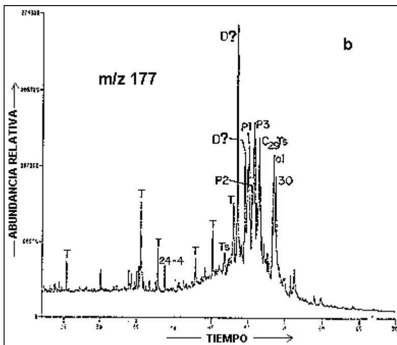
Distribución de biomarcadores terpanos m/z 191(a) y m/z 177(b) del mene Quirós (Tomado de: Del Olio, 1993)
