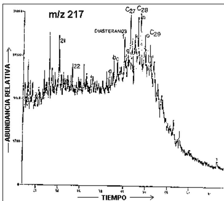
Distribución de biomarcadores esteranos m/z 217 del mene Quirós (Tomado de: Del Olio, 1993)
